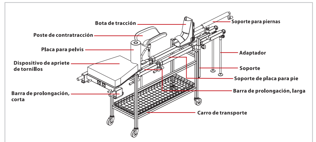
Extensión para ortopedia 115-005691-00&115-005780-00 (carro de transporte)
